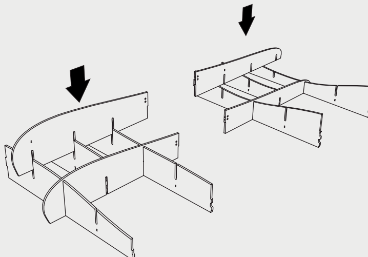
Obere Möbelhälften
