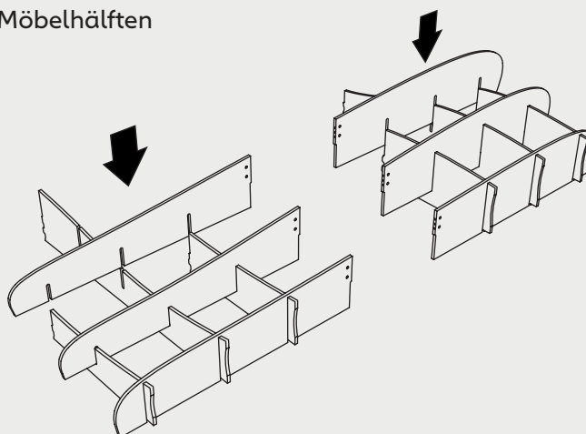
Obere Möbelhälften
